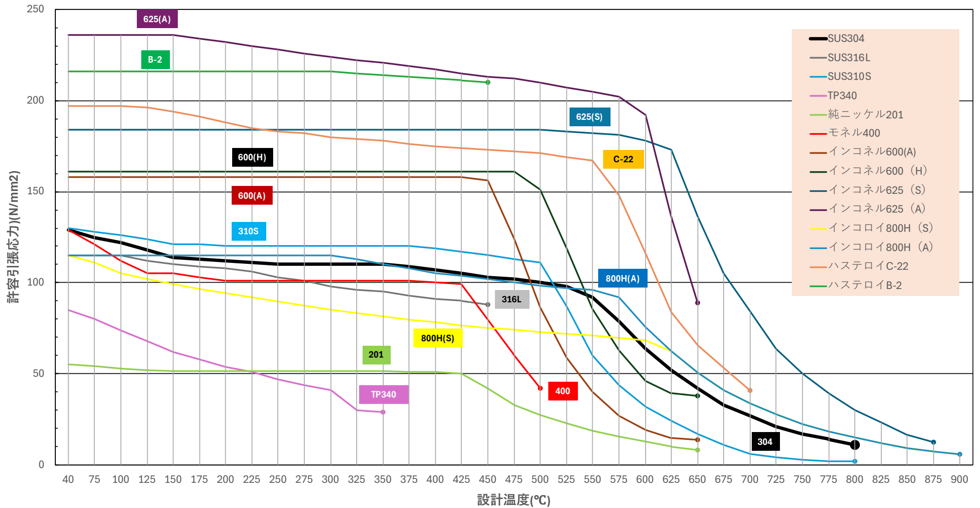
材料の設計温度における許容引張応力(N/mm 2 )
